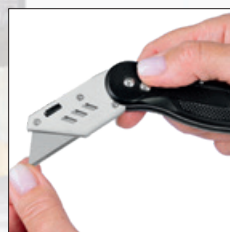
Feststellmechanismus
